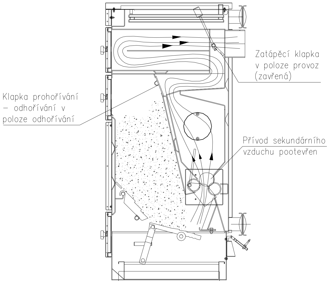
Obr. 6 Řez kotlem při způsobu spalování paliva odhoříváním
