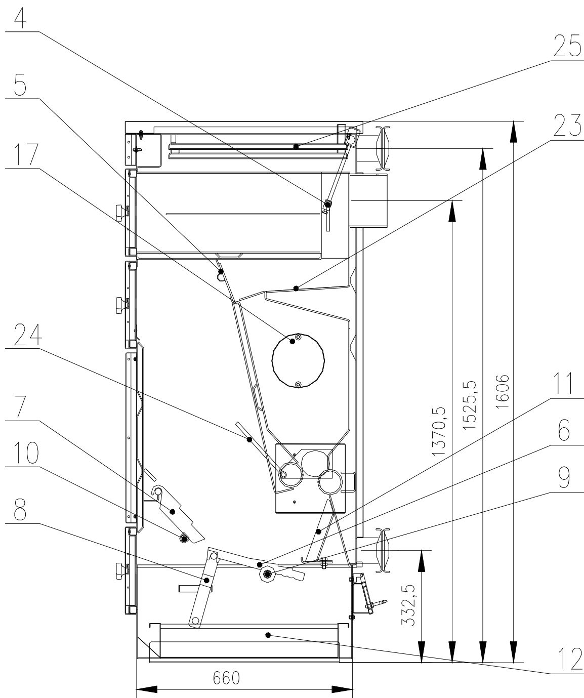
Obr. 3 Řez kotlem
