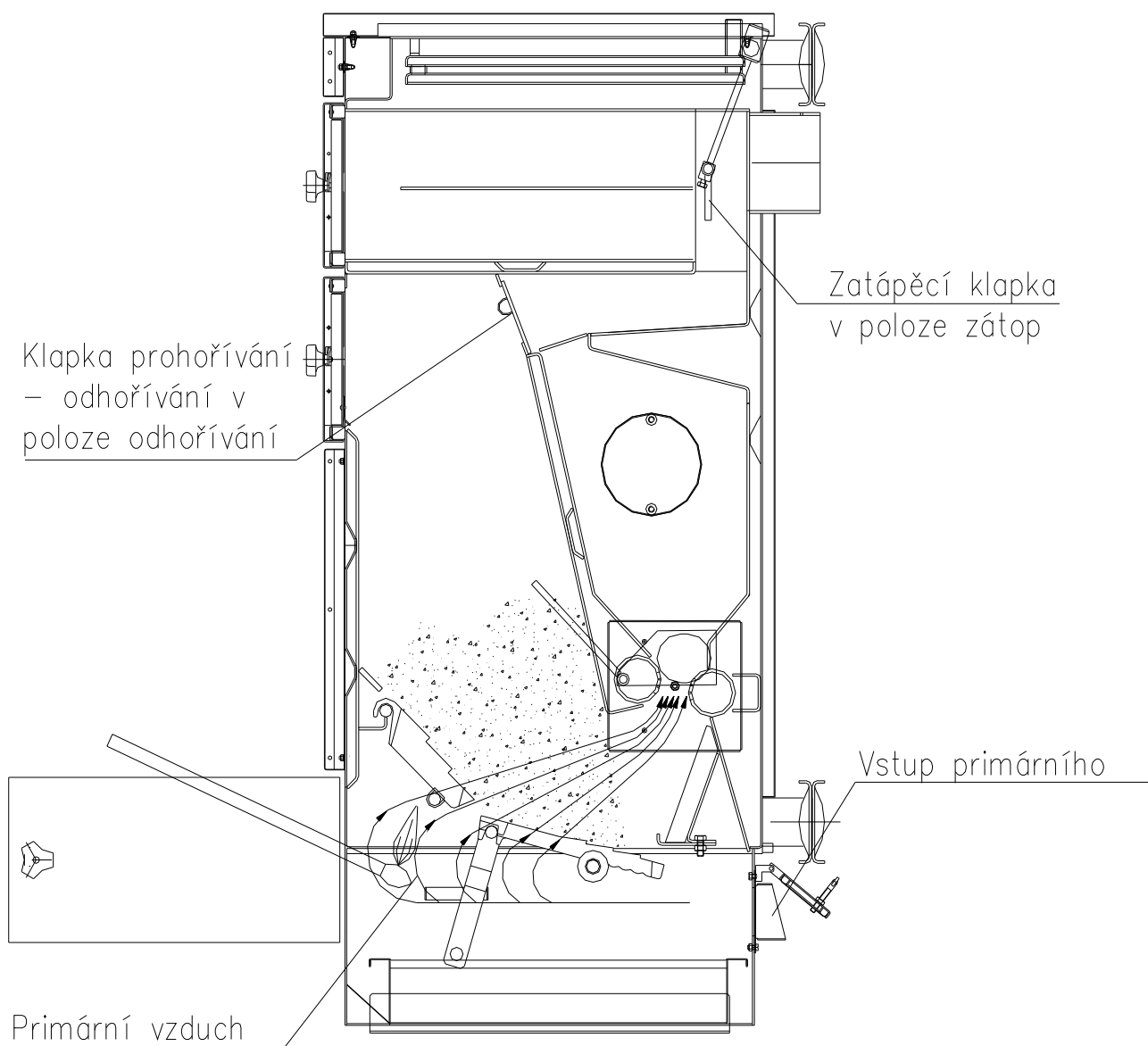
Obr. 5 Řez kotlem při zatápění
