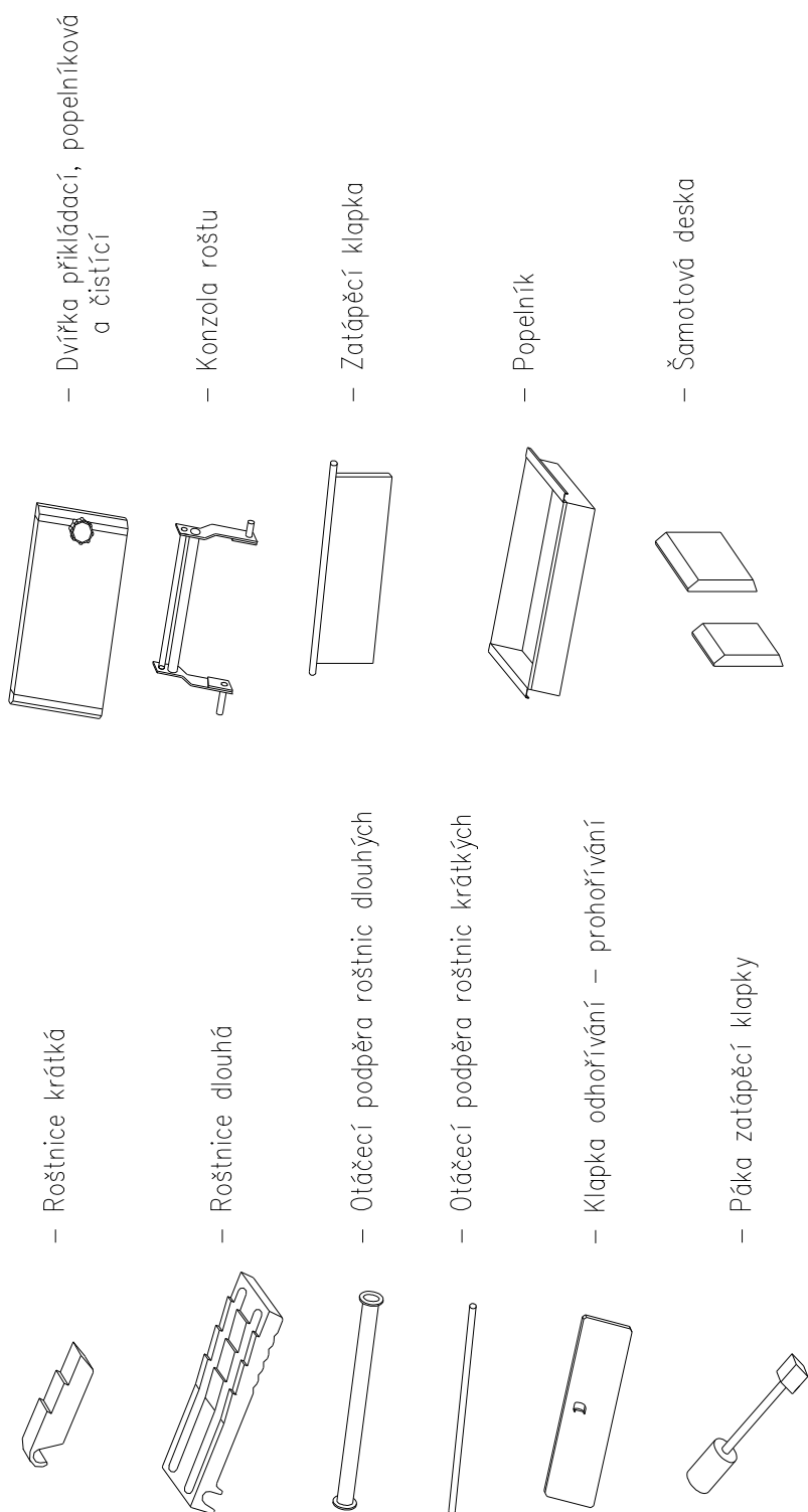
obr. 2 Vybrané náhradní díly pro kotle H 635 a H650
