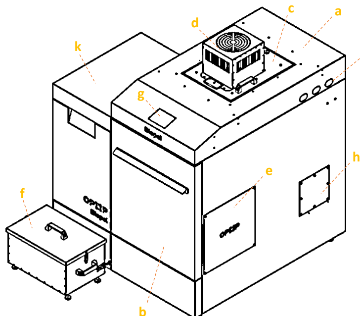
Biopel set s kompaktní násypkou na pelety
